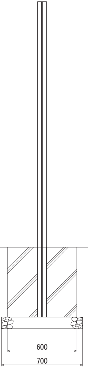
【側面図 S=1:20】
