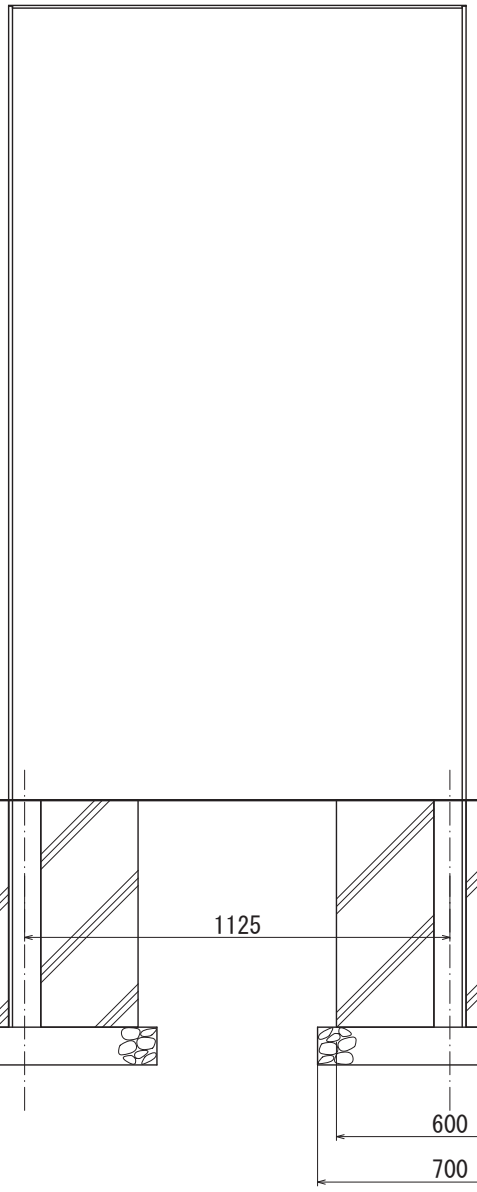
【正面図 S=1:20】
