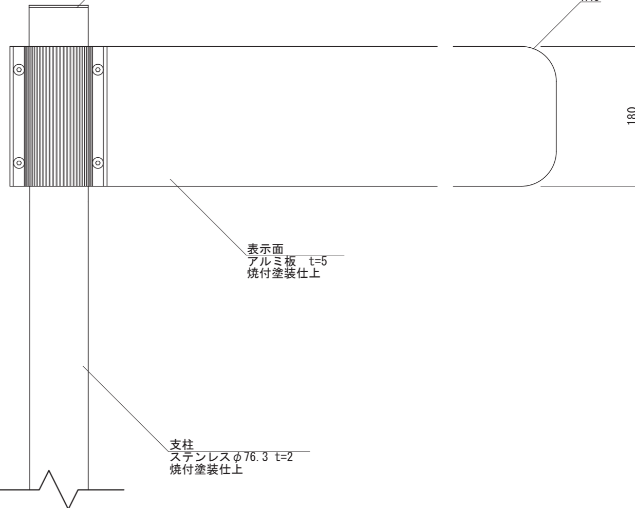
【正面図 S=1:5】
