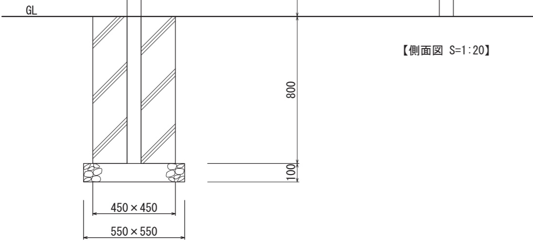
【正面図 S=1:20】
