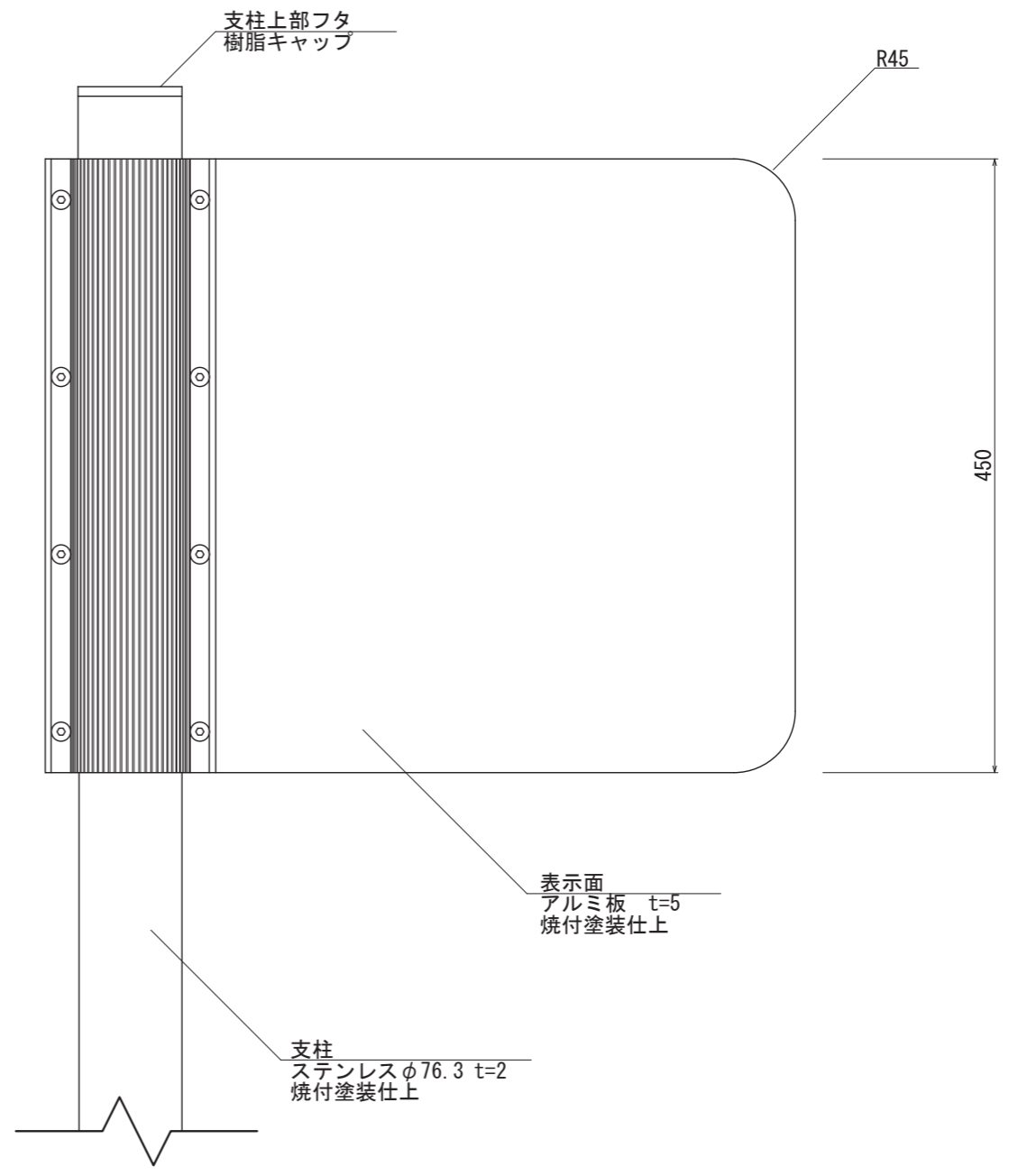
【正面図 S=1:5】
