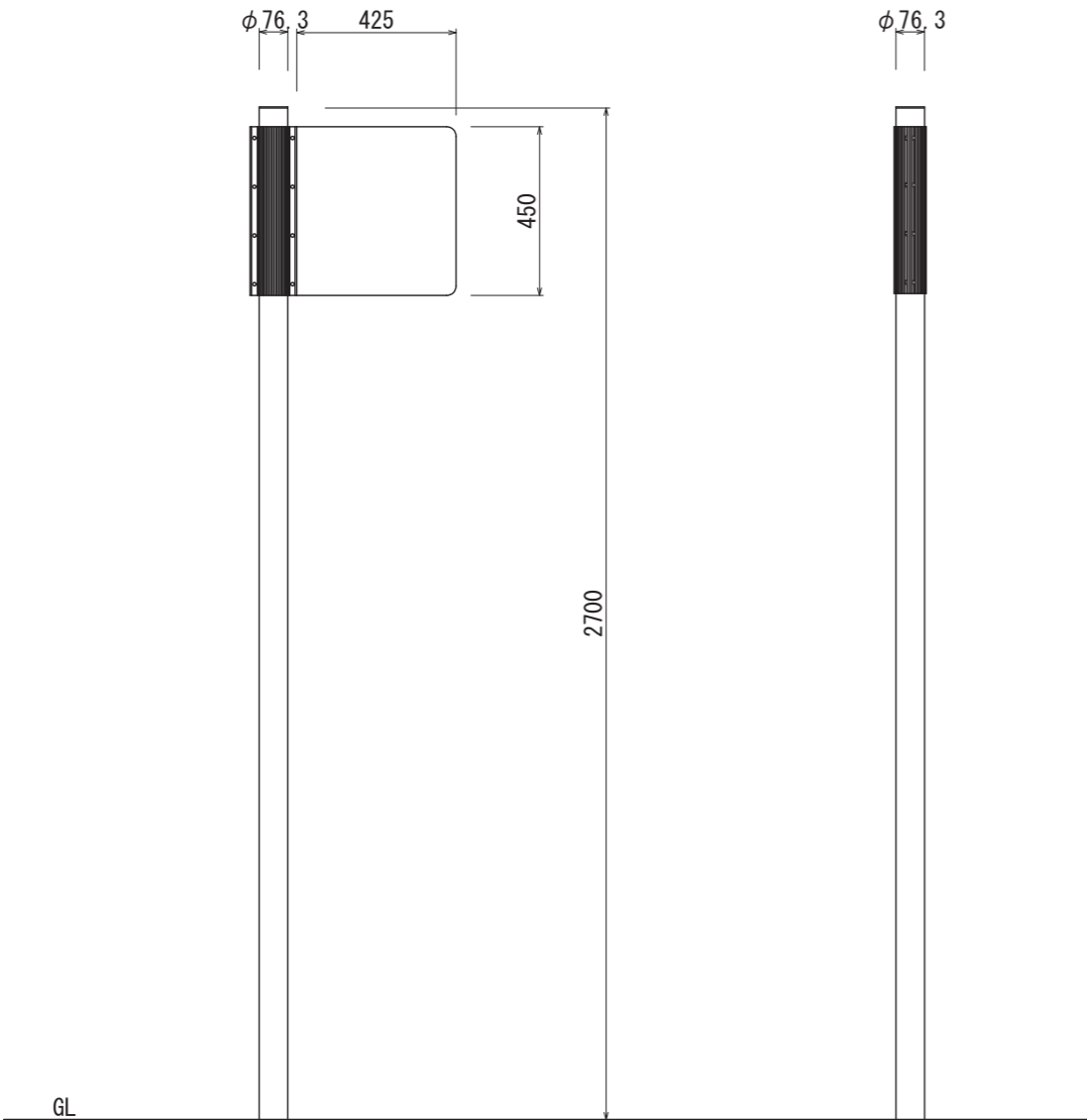
【側面図 S=1:20】
