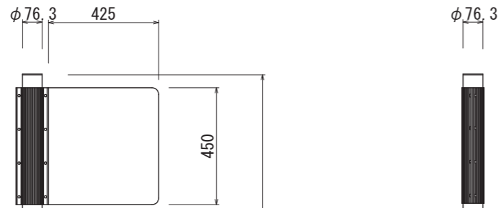
【平面図 S=1:20】
