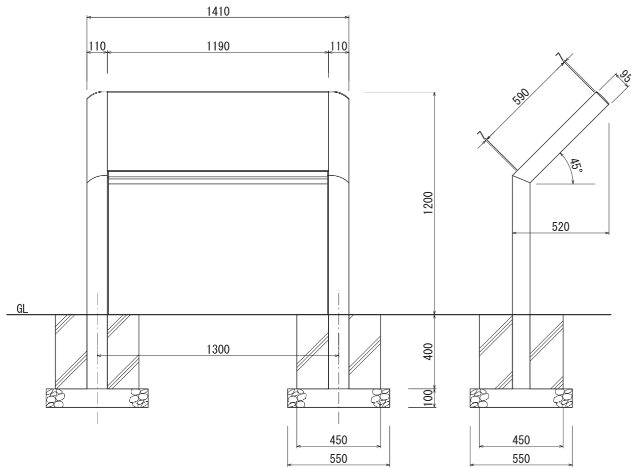
【側面図 S=1:20】
