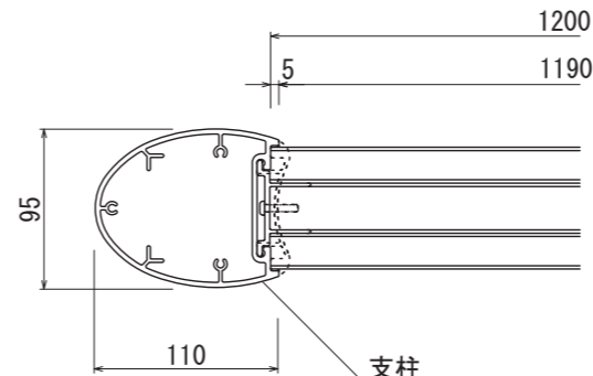
【平面図 S=1:5】
