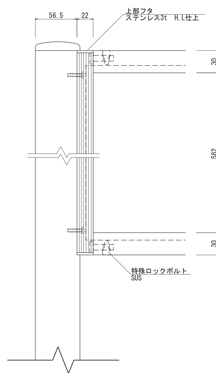
【正面図 S=1:3】
