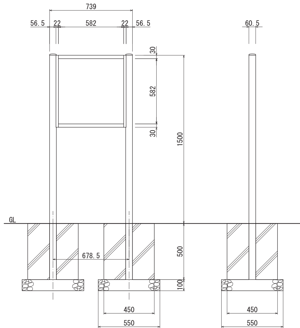
【正面図 S=1:20】
