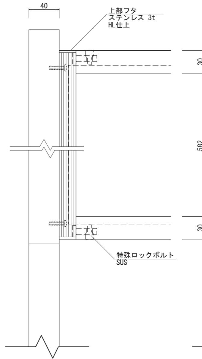
【正面図 S=1:3】
