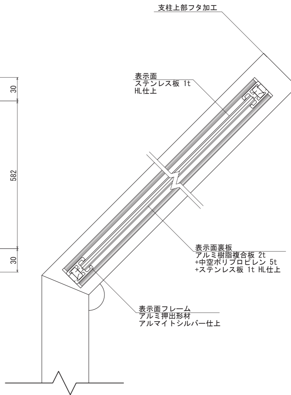
【側断面図 S=1:3】
