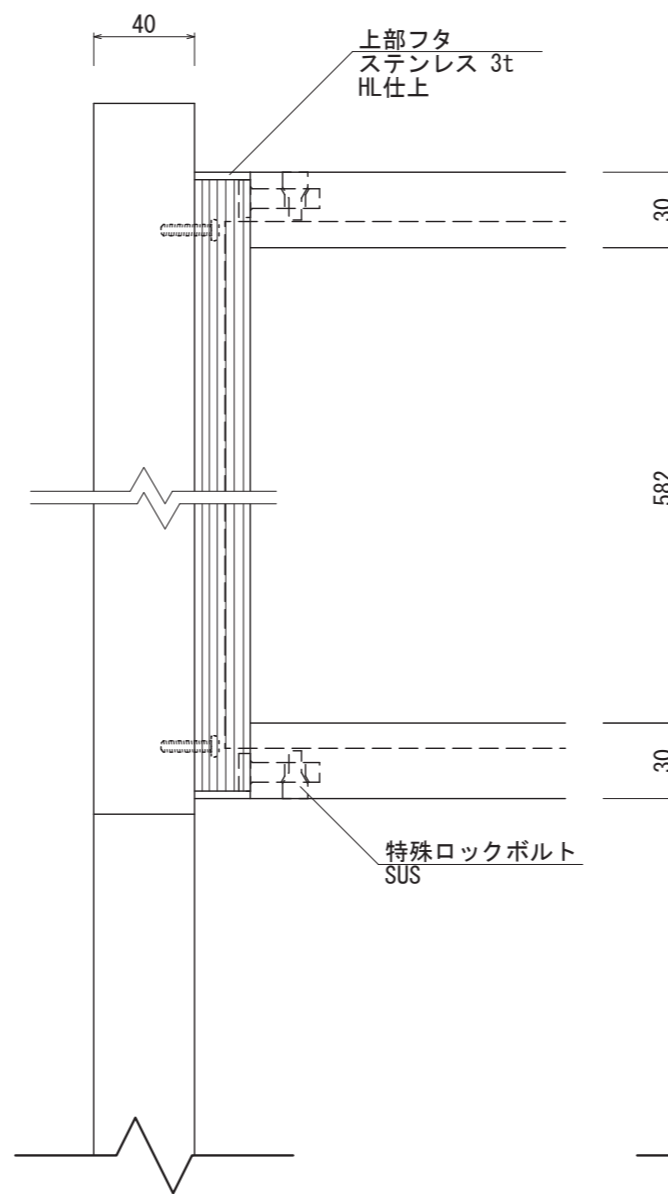
【正面図 S=1:3】
