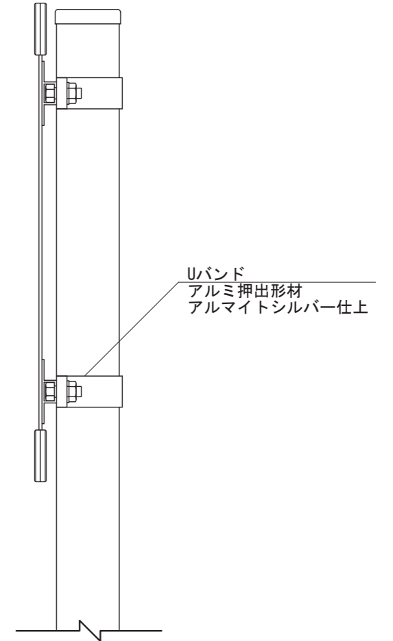
【側面図 S=1:5】
