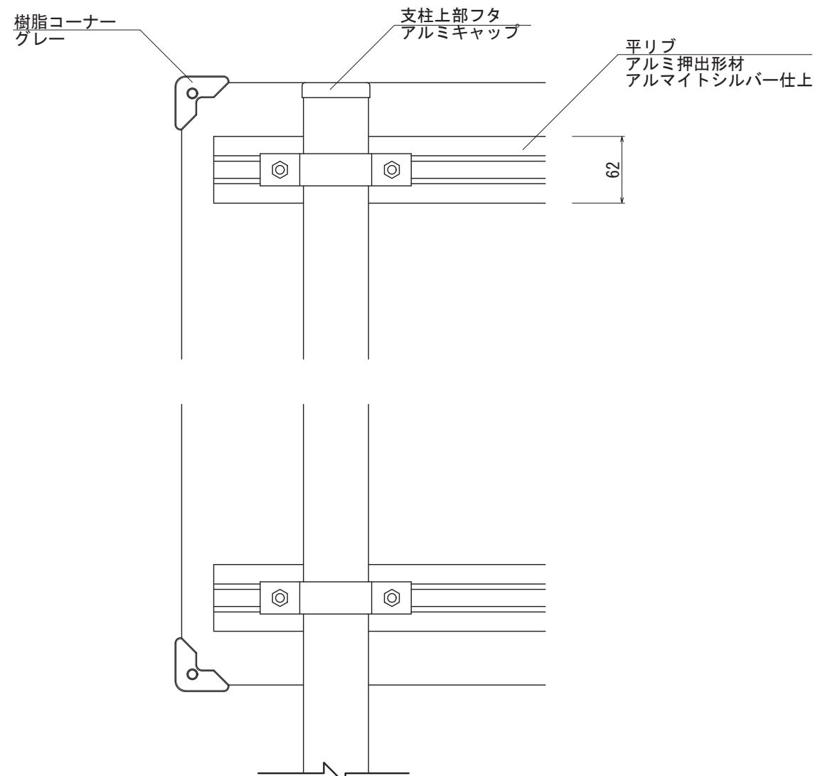
【背面図 S=1:5】
