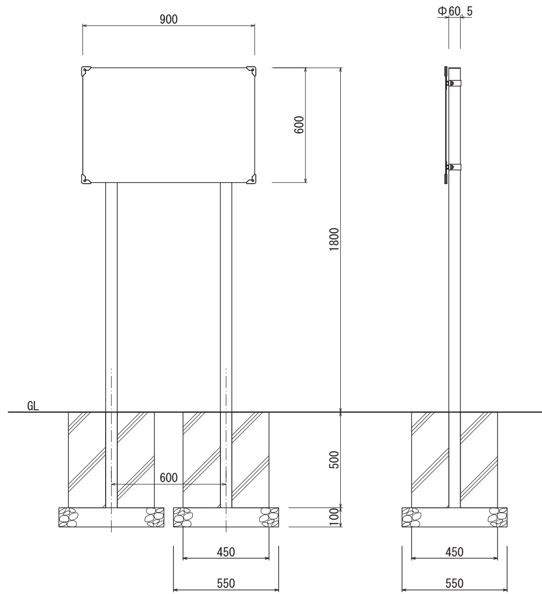
【正面図 S=1:20】
