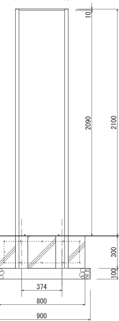
【正面図 S=1:20】
