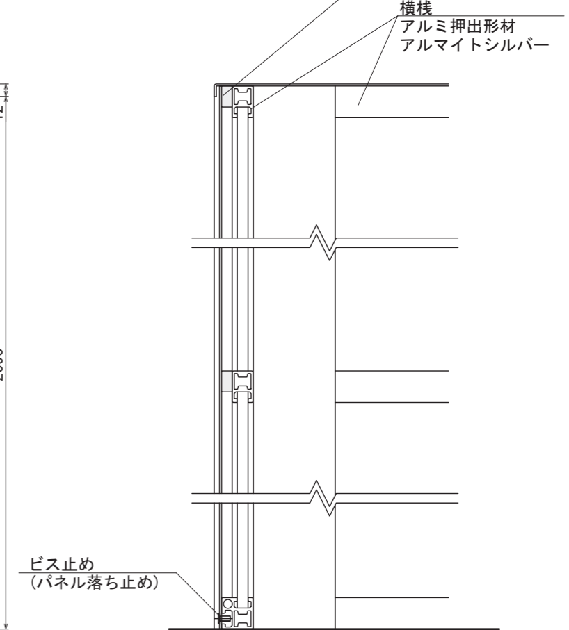
【断面図 S=1:5】
