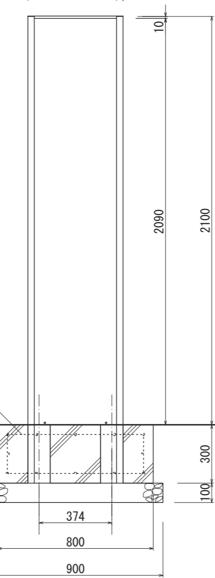
【側面図 S=1:20】
