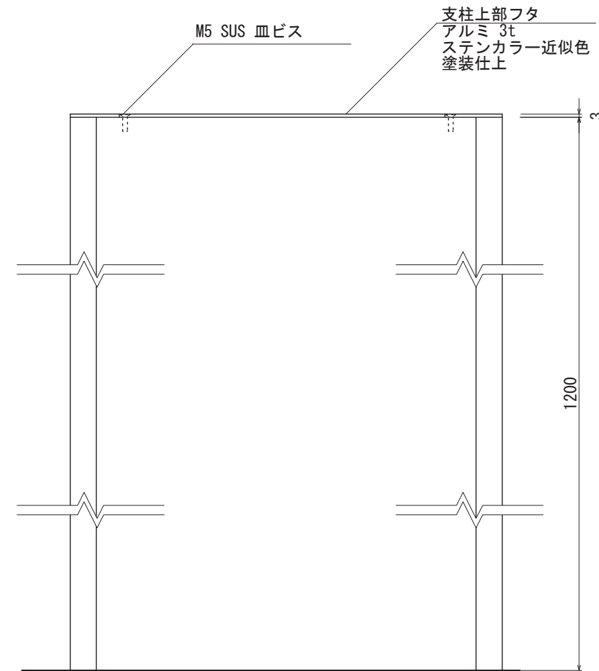
【正面図 S=1:5】
