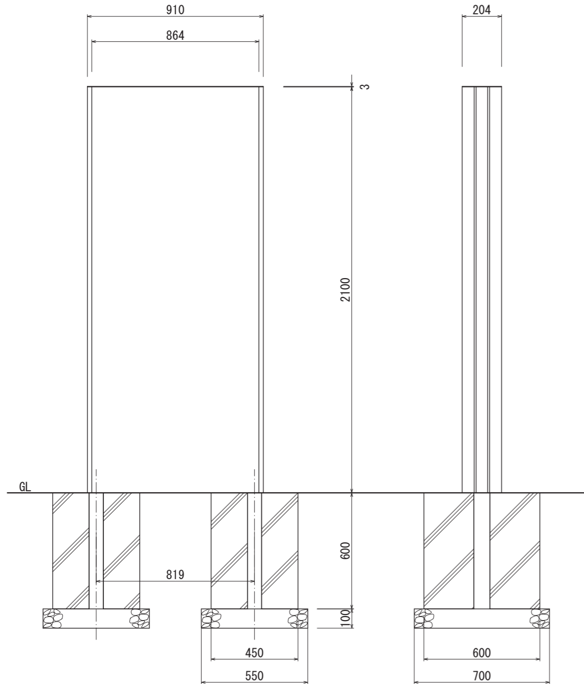
【正面図 S=1:20】
