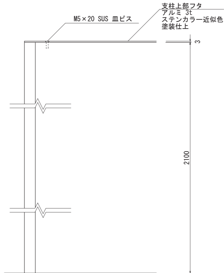
【正面図 S=1:5】
