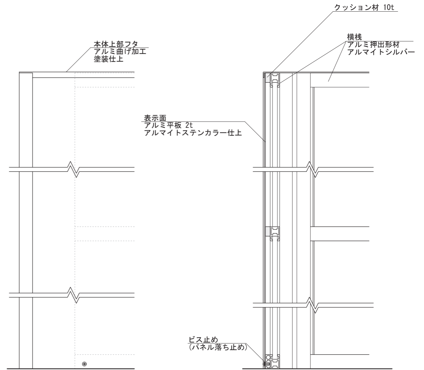
【断面図 S=1:5】
