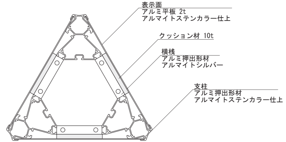
【断面図 S=1:5】
