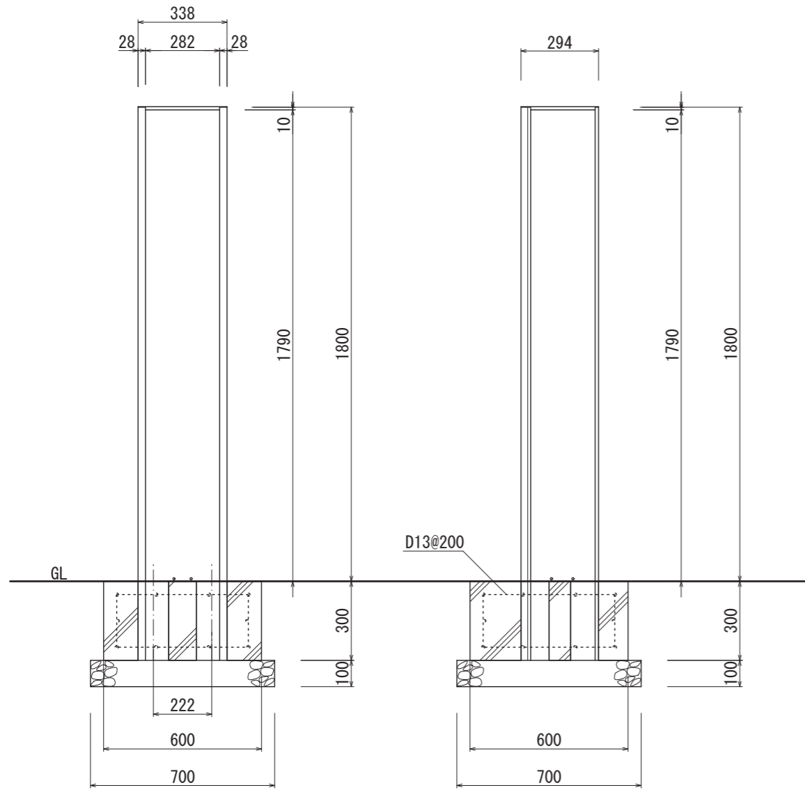
【正面図 S=1:20】
