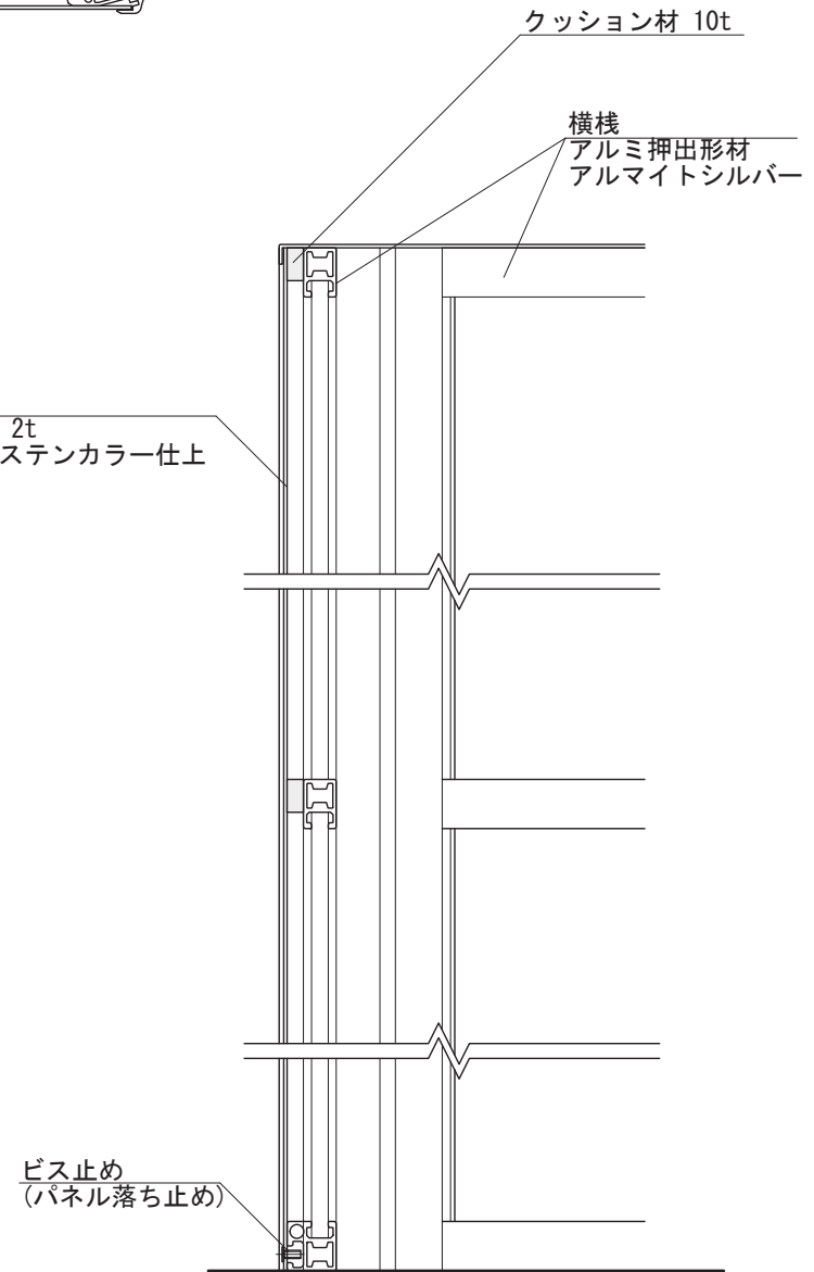
【断面図 S=1:5】
