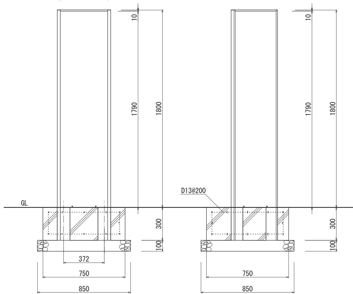
【正面図 S=1:20】
