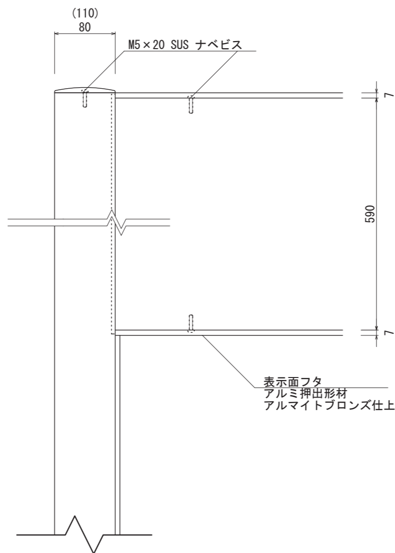
【正面図 S=1:5】
