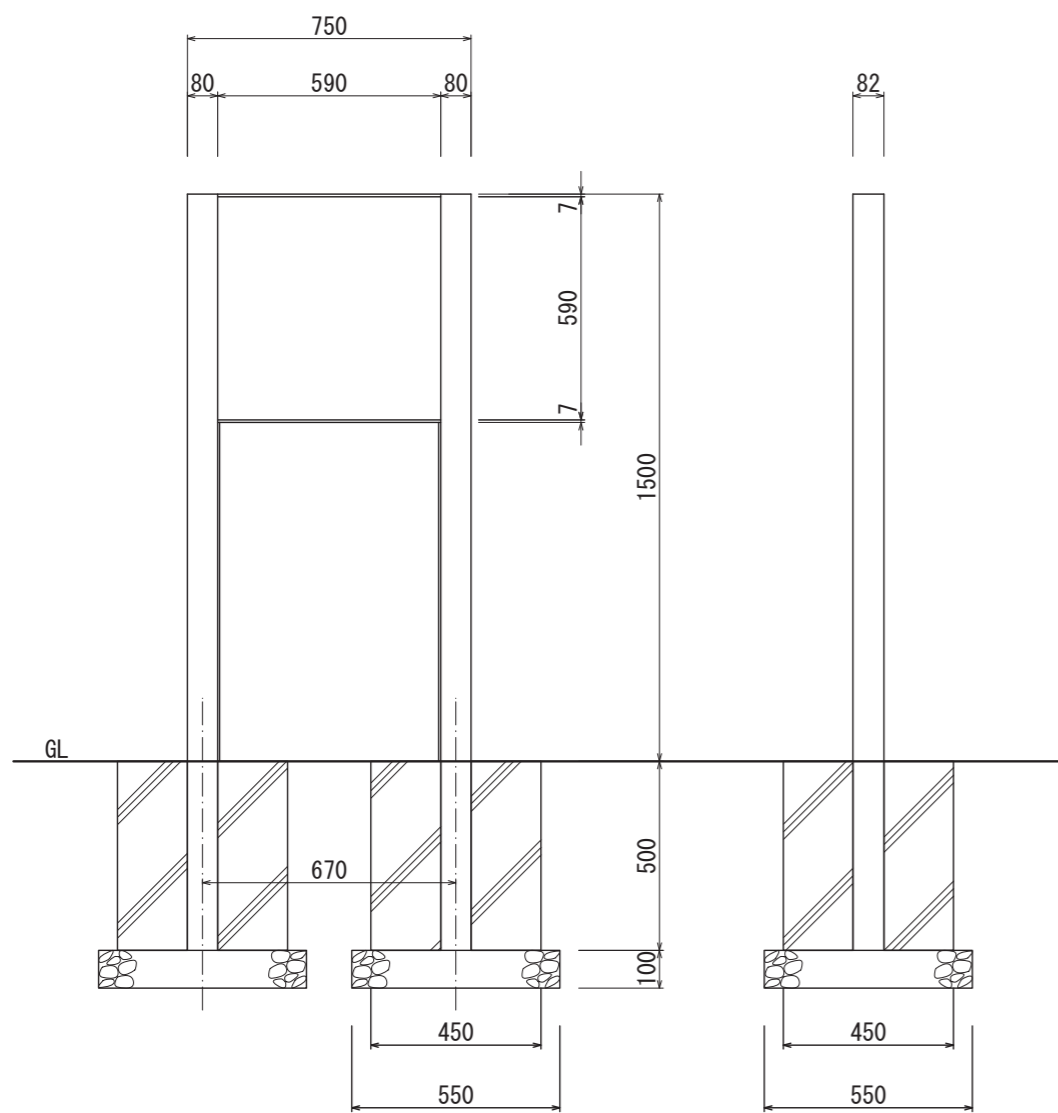
【正面図 S=1:20】
