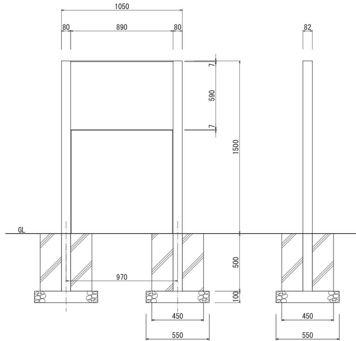
【正面図 S=1:20】
