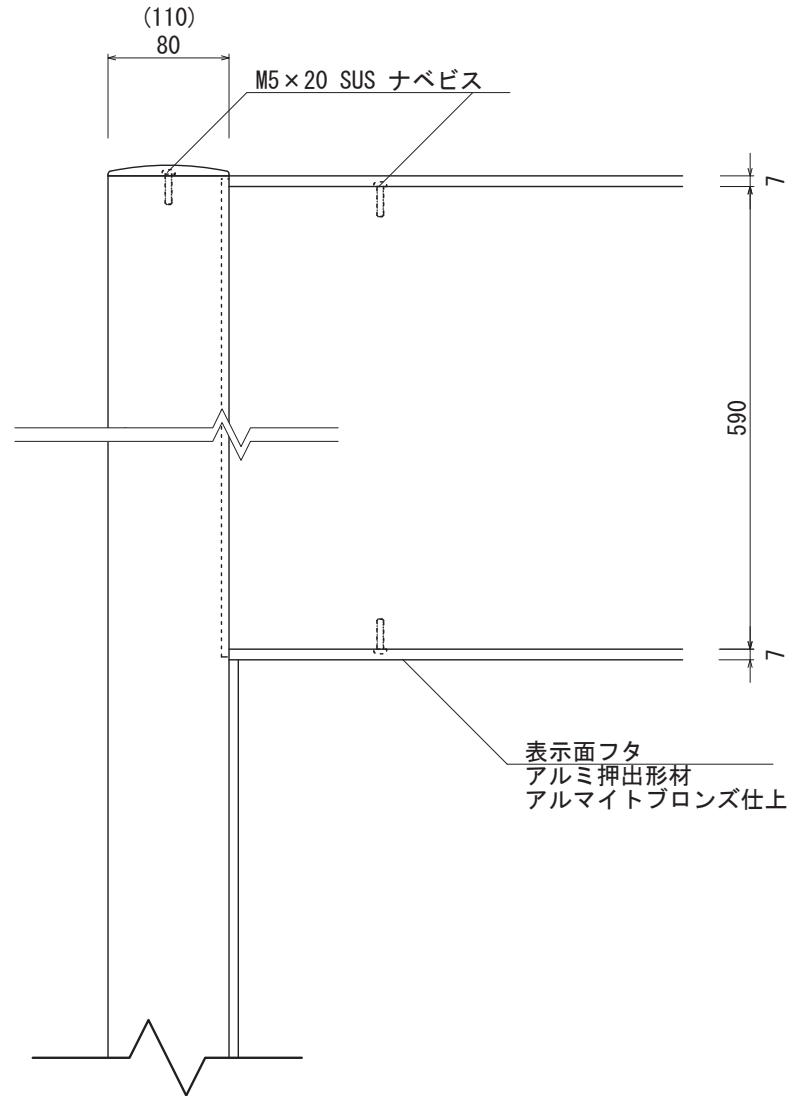
【正面図 S=1:5】
