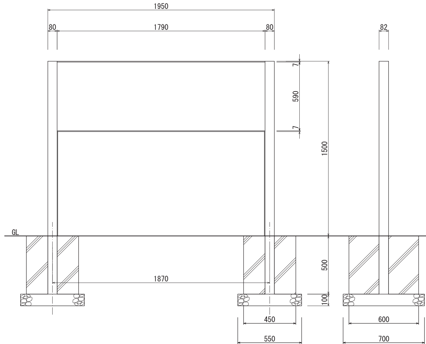
【正面図 S=1:20】
