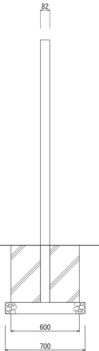
【側面図 S=1:20】
