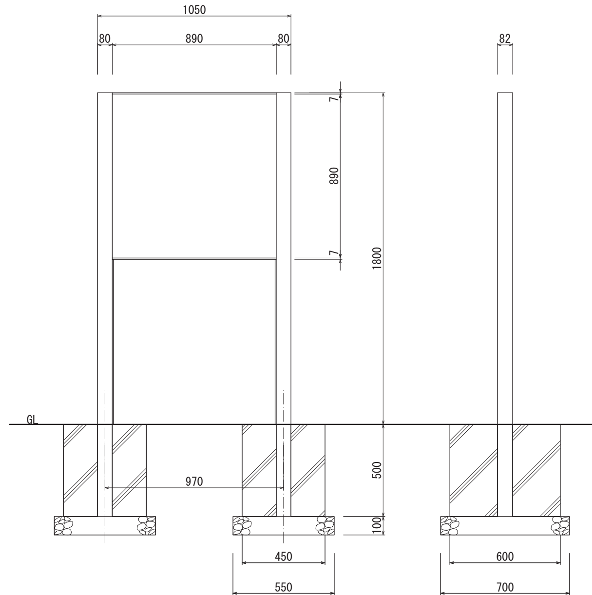
【正面図 S=1:20】
