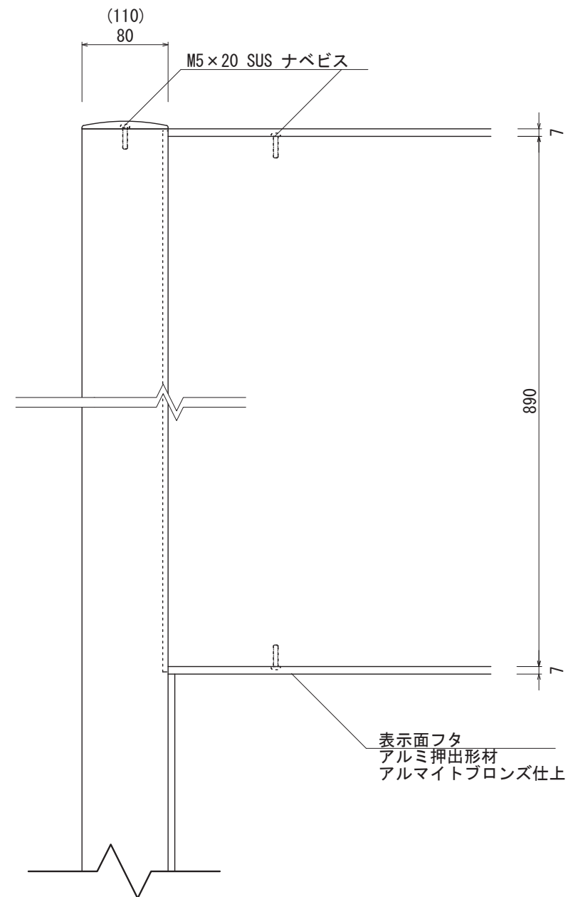
【正面図 S=1:5】
