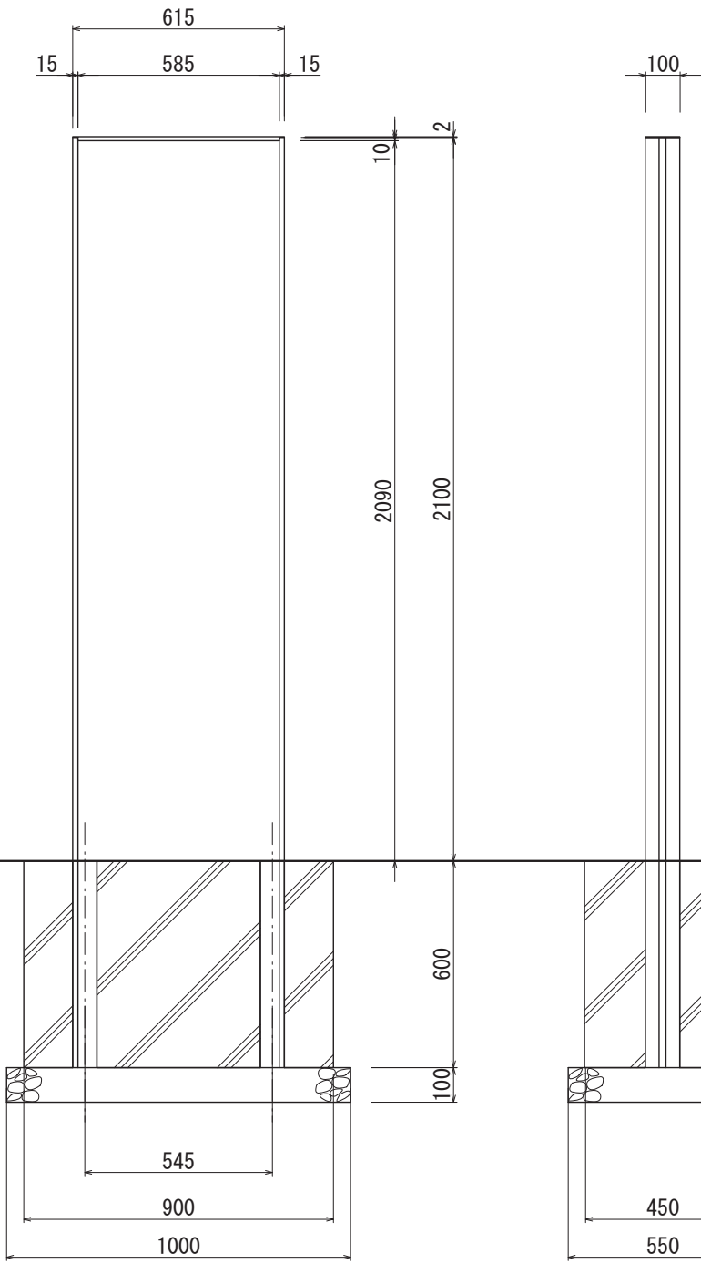
【正面図 S=1:20】
