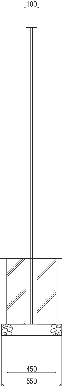
【側面図 S=1:20】
