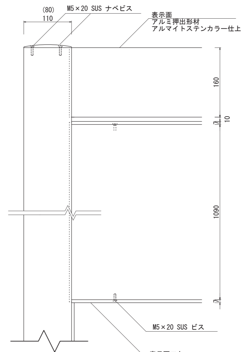
【正面図 S=1:5】
