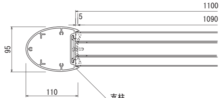
【平面図 S=1:5】
