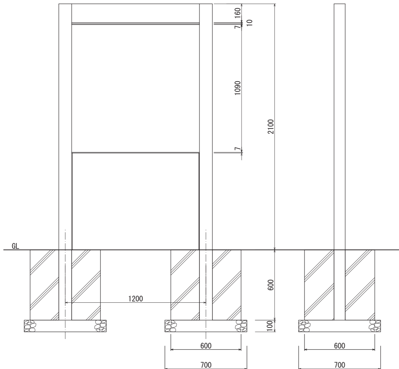
【正面図 S=1:20】
