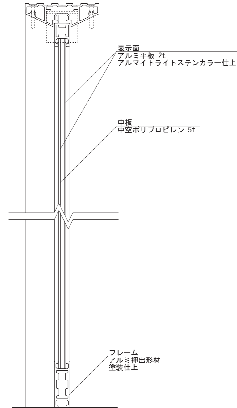
【側面図 S=1:3】
