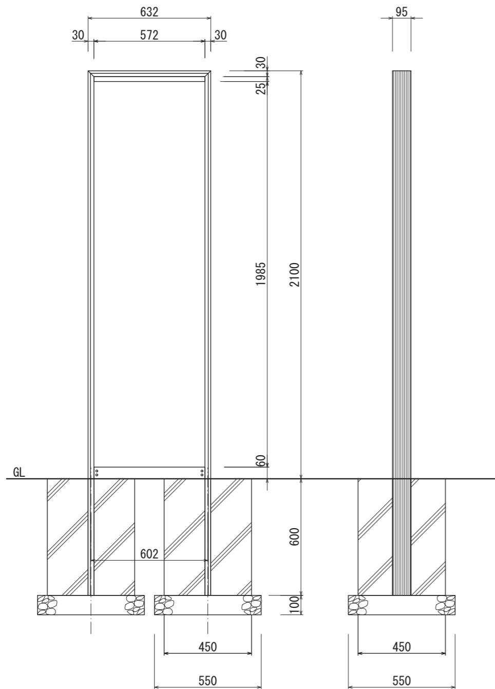
【正面図 S=1:20】
