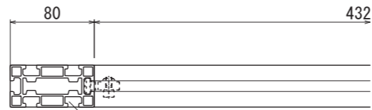
【平面図 S=1:5】
