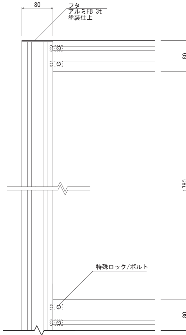
【正面図 S=1:5】
