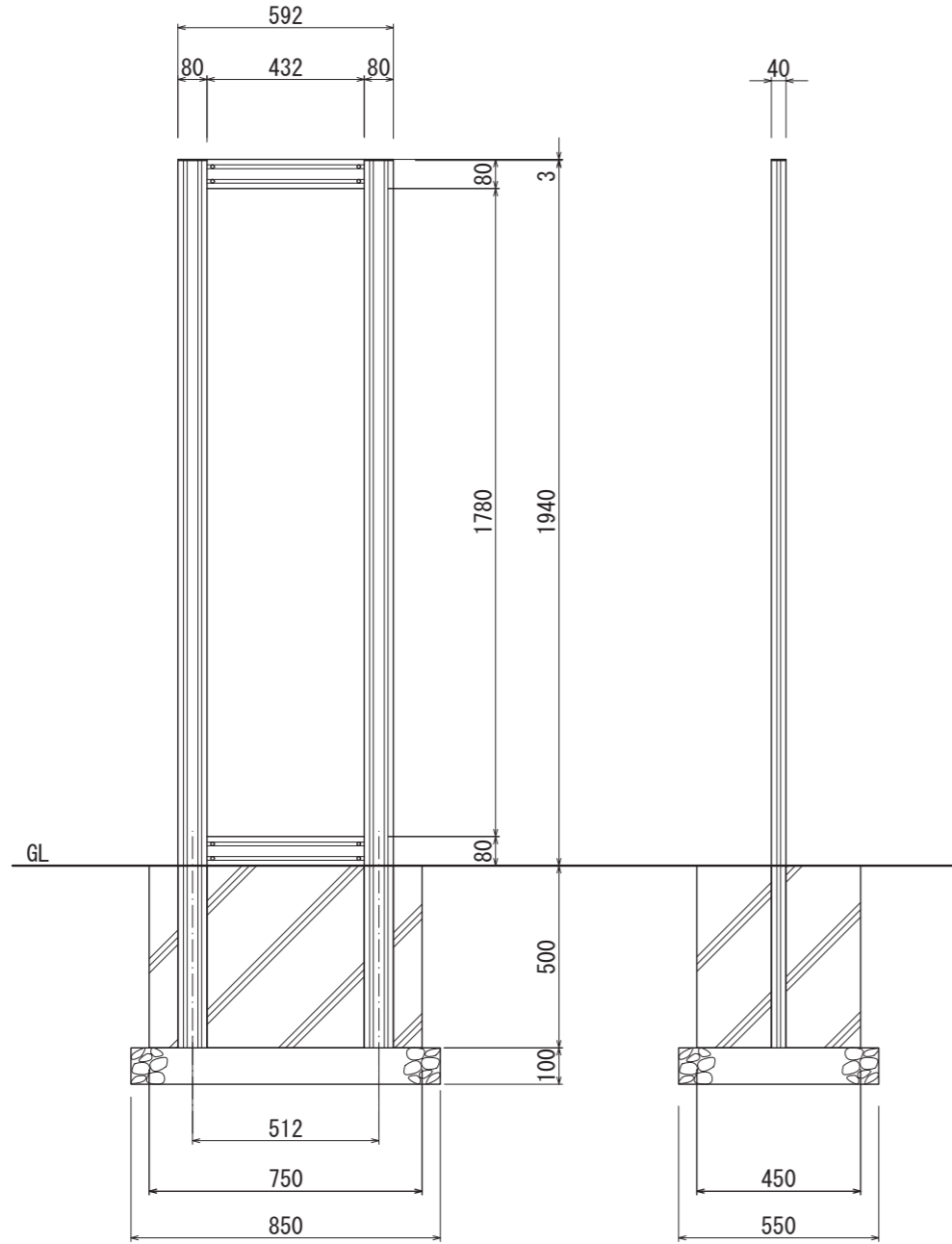
【正面図 S=1:20】
