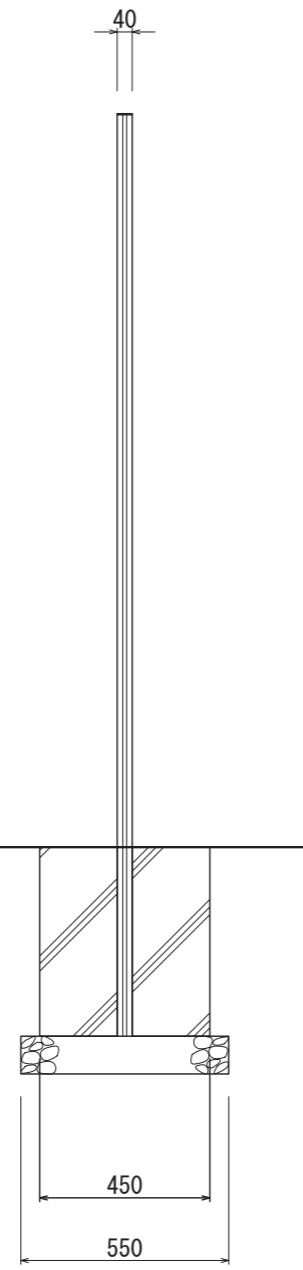
【側面図 S=1:20】
