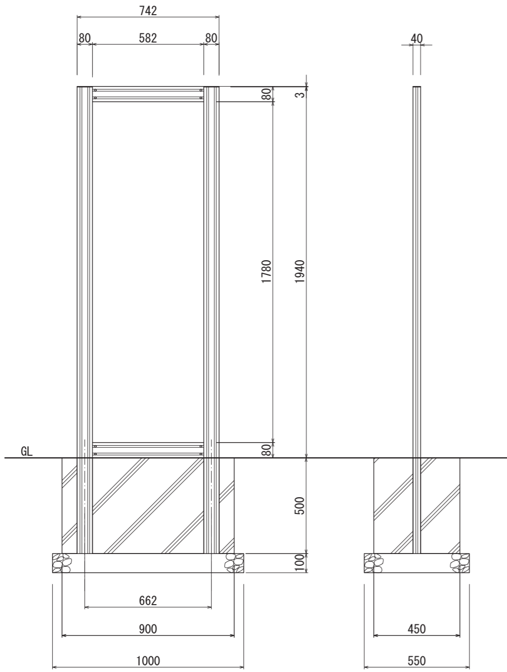
【正面図 S=1:20】
