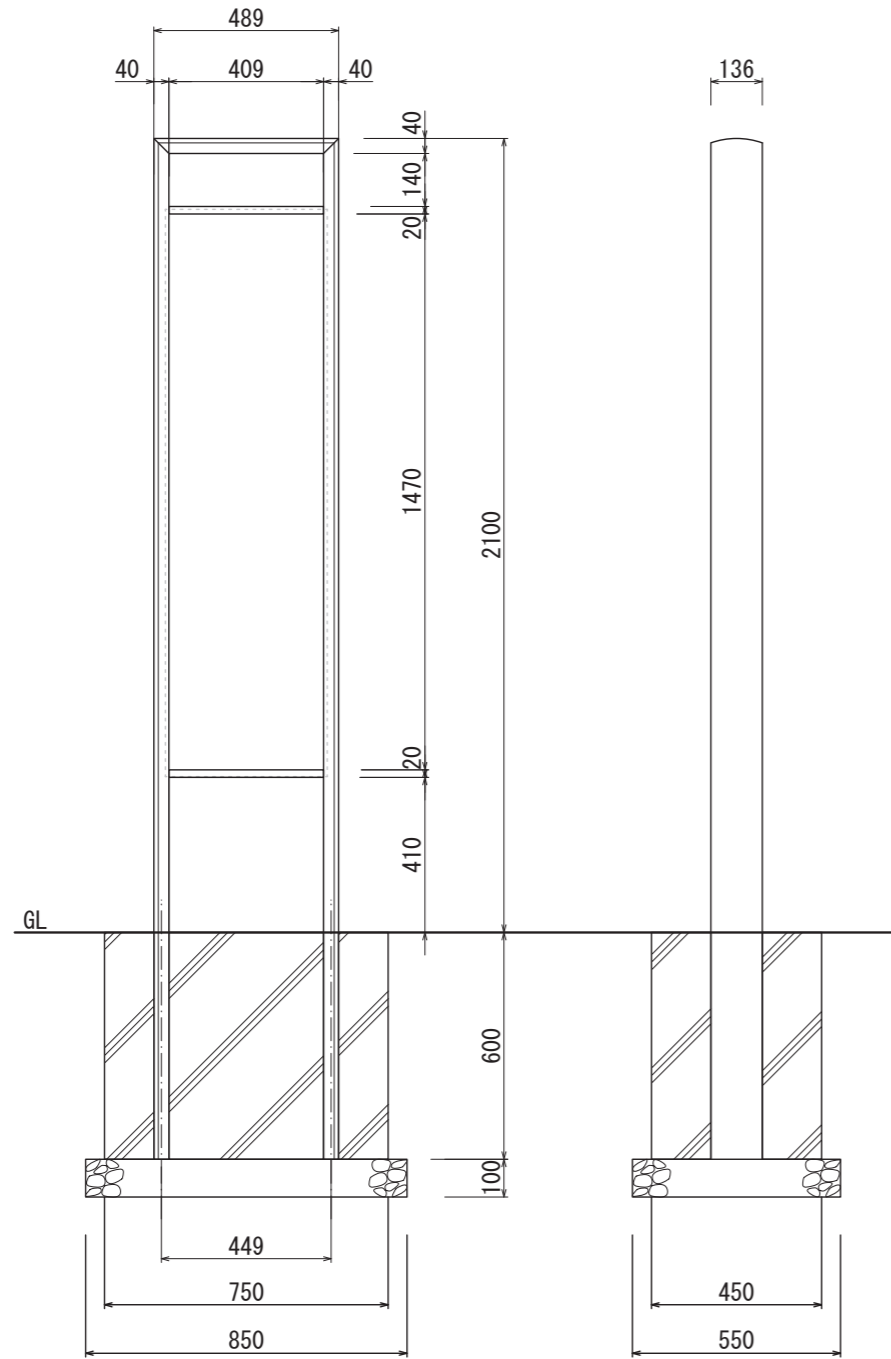
【正面図 S=1:20】
