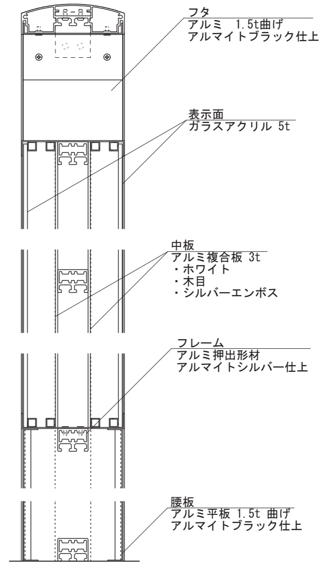
【側面図 S=1:5】
