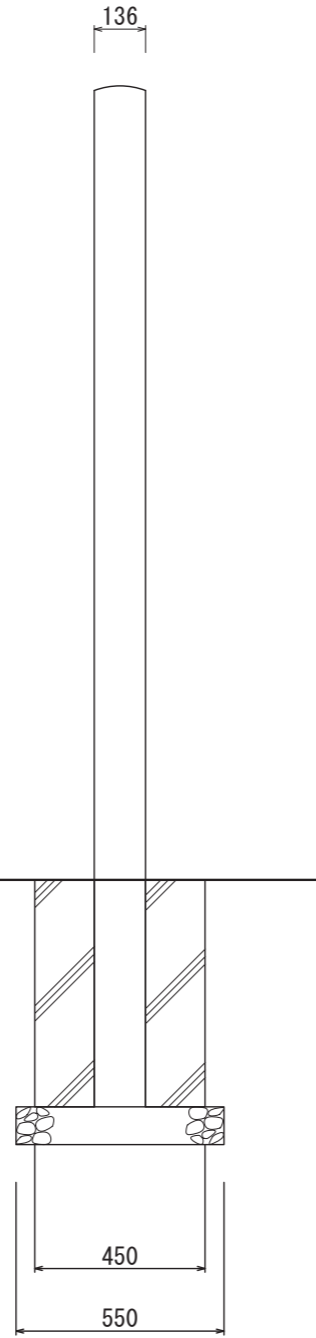
【側面図 S=1:20】
