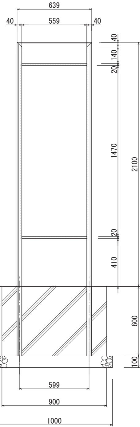
【正面図 S=1:20】
