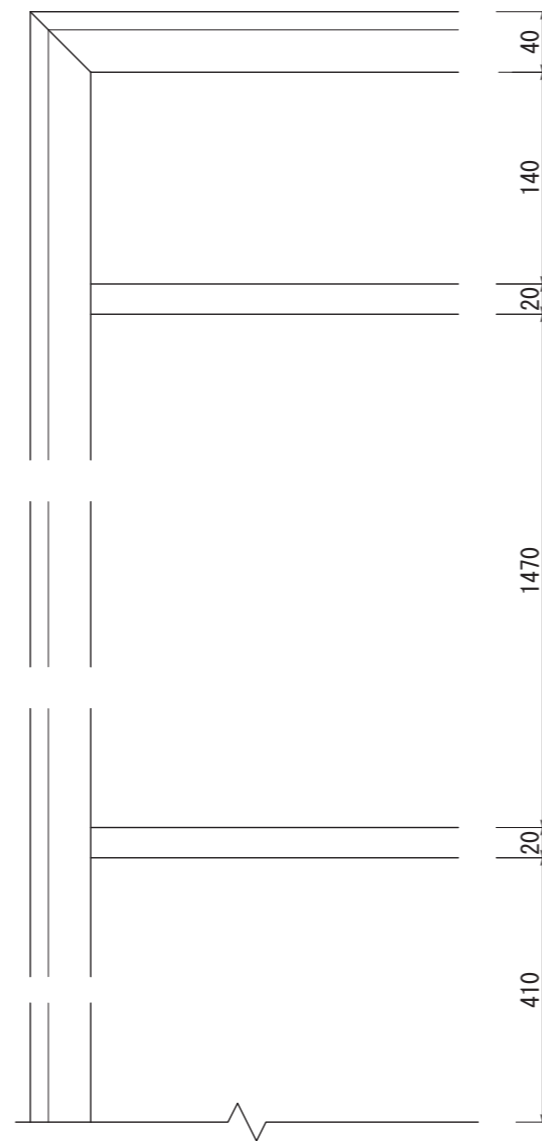
【正面図 S=1:5】
