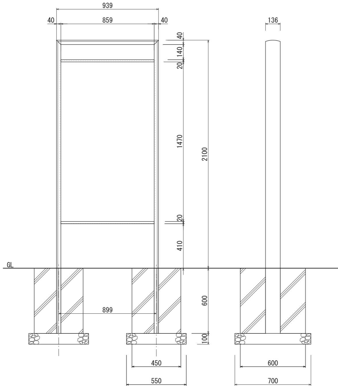
【正面図 S=1:20】
