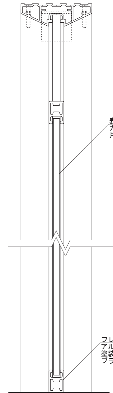
【側面図 S=1:3】
