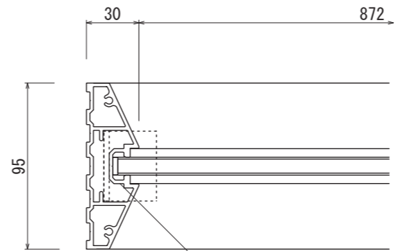
【平面図 S=1:3】
