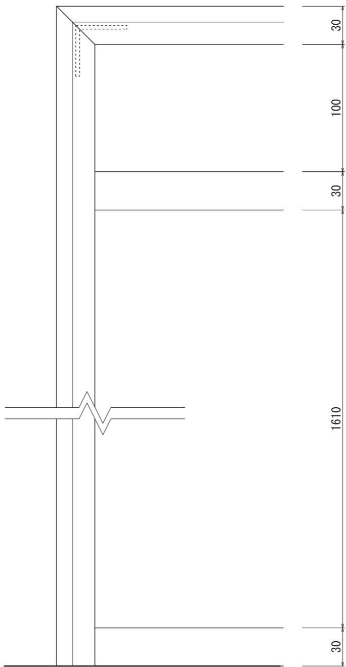
【正面図 S=1:3】
