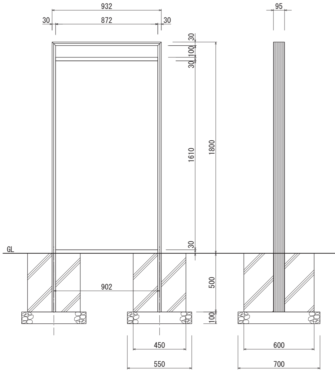
【正面図 S=1:20】
