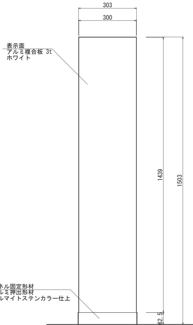
【正面図 S=1:10】
