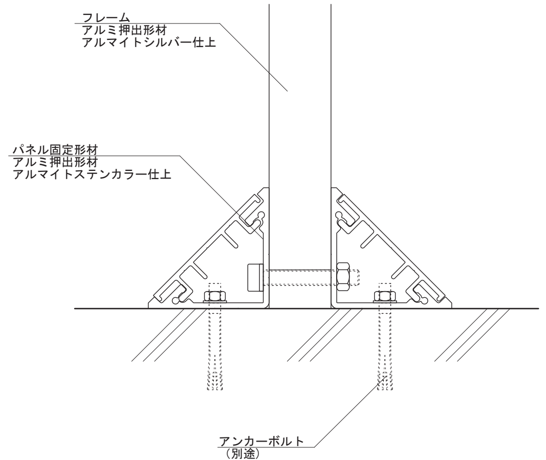
【断面図 S=1:2】
