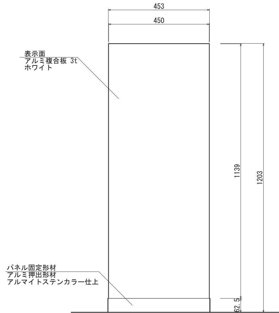
【正面図 S=1:10】
