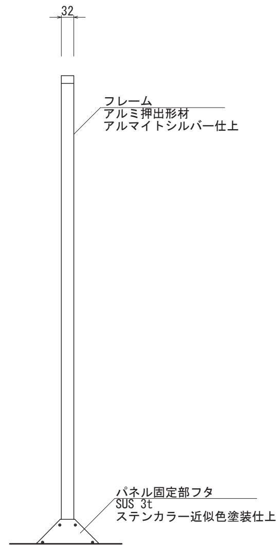
【側面図 S=1:10】
