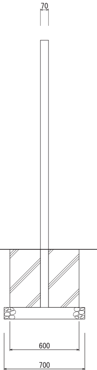
【側面図 S=1:20】
