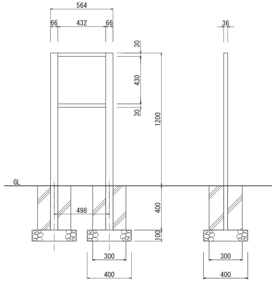
【正面図 S=1:20】
