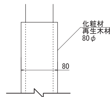
【背面図 S=1:5】
