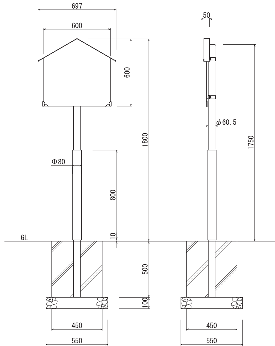
【正面図 S=1:20】
