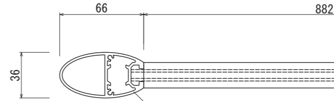
【平面図 S=1:3】
