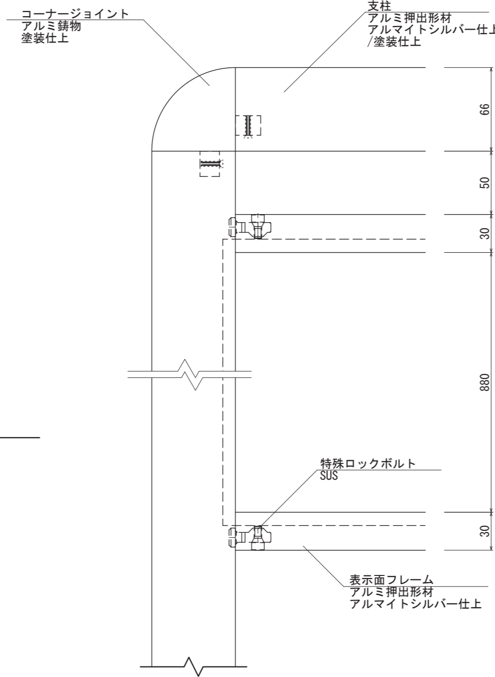
【正面図 S=1:3】
