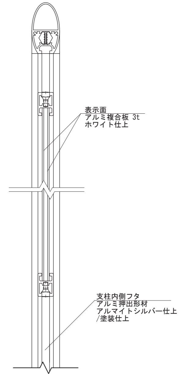
【側面図 S=1:3】
