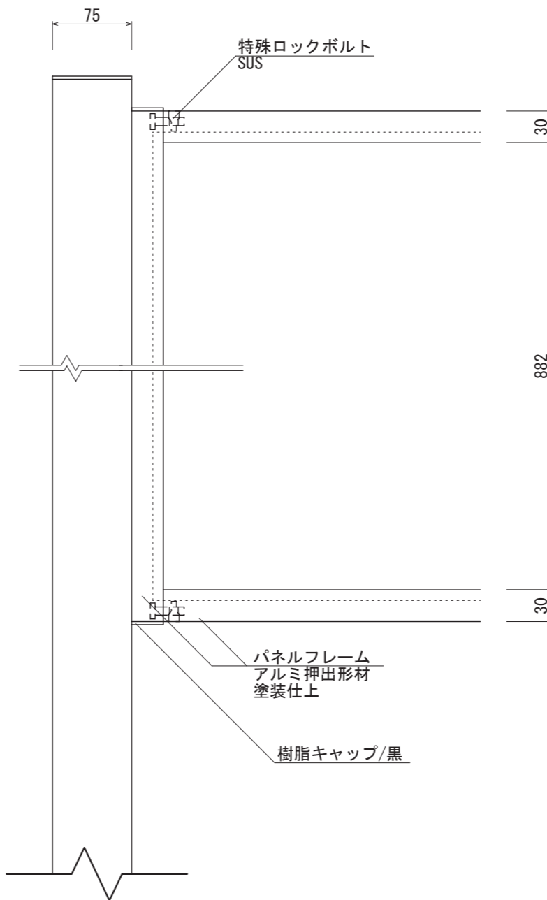
【正面図 S=1:5】
