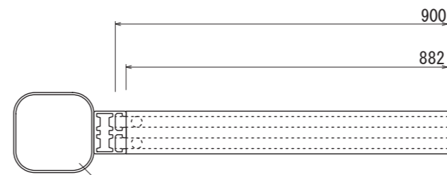
【平面図 S=1:5】
