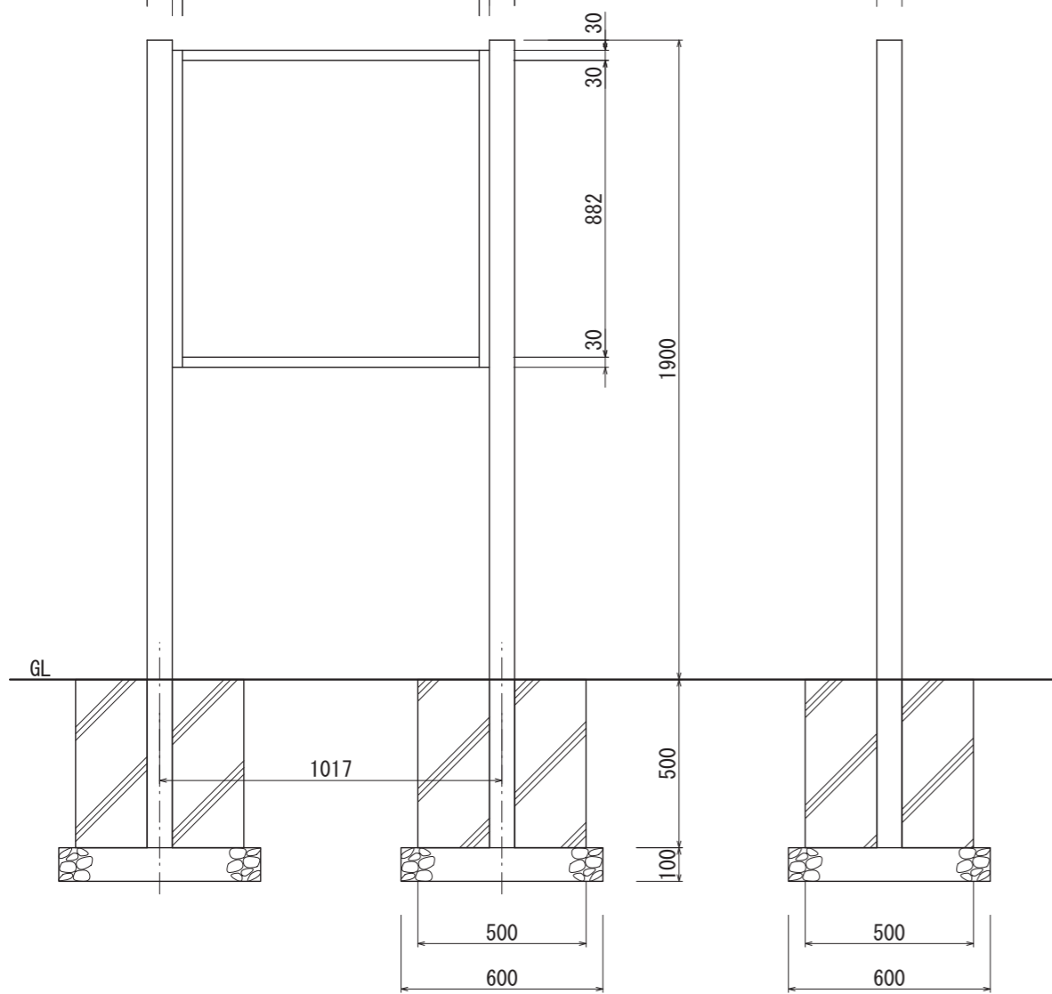
【正面図 S=1:20】
