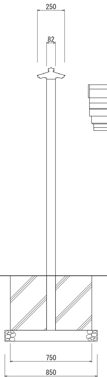
【側面図 S=1:20】
