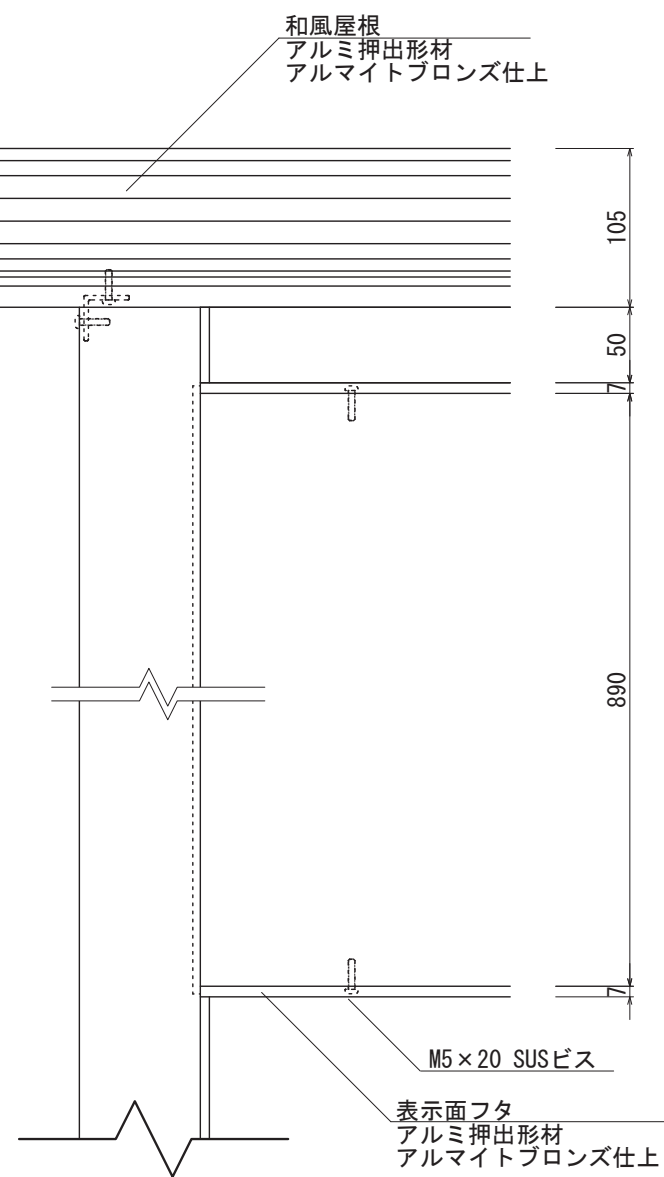
【正面図 S=1:5】
