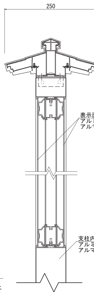
【側断面図 S=1:5】
