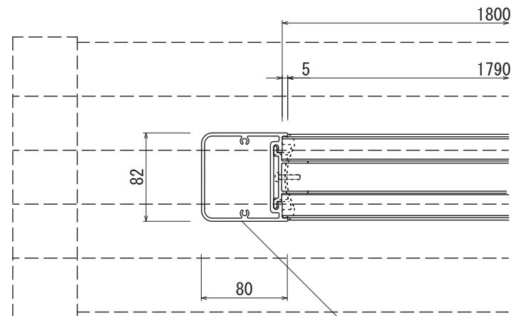
【平面図 S=1:5】
