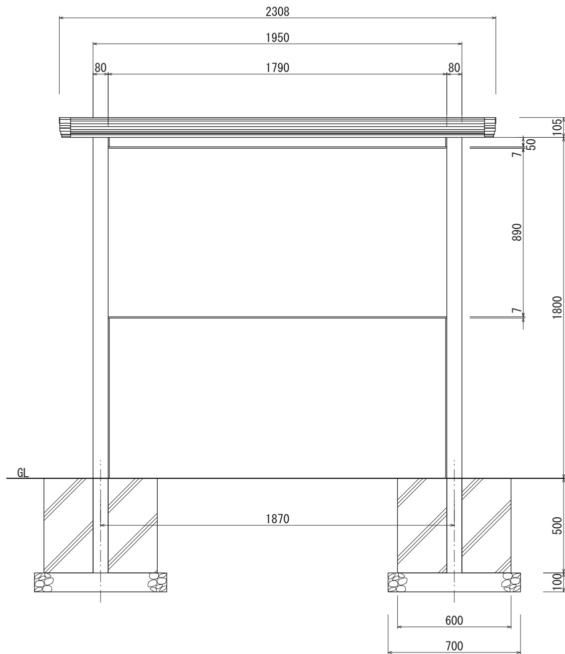
【正面図 S=1:20】
