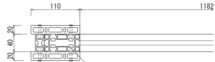
【平面図 S=1:5】
