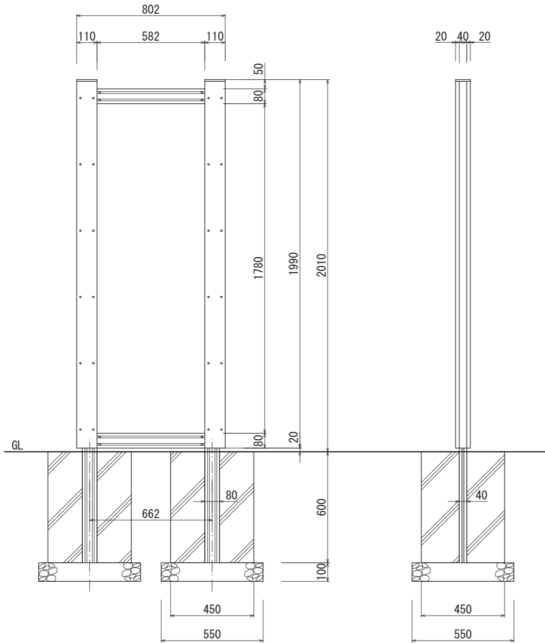
【正面図 S=1:20】
