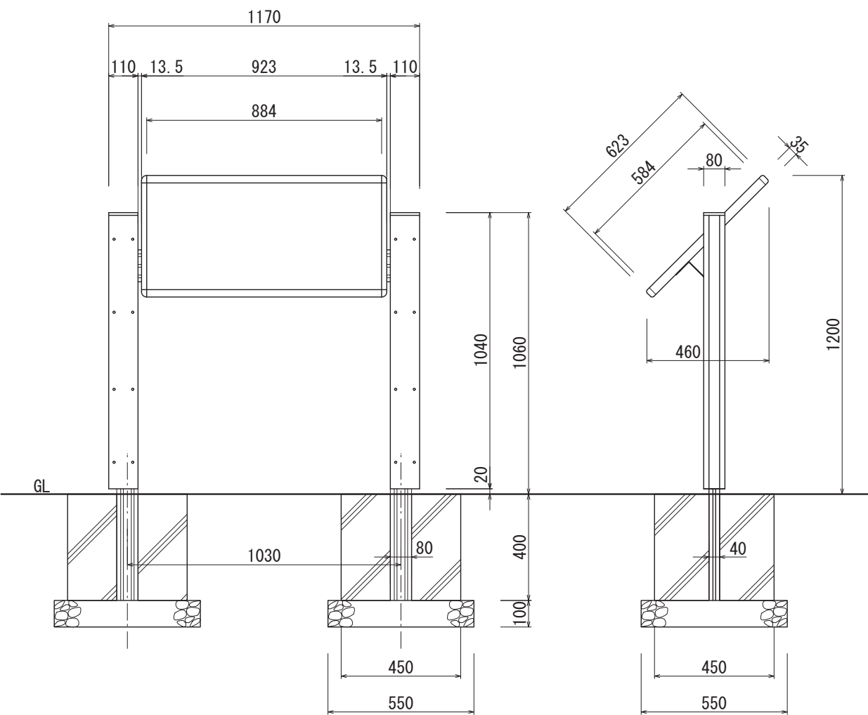
【正面図 S=1:20】
