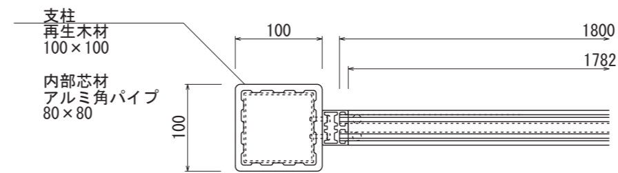
【平面図 S=1:5】
