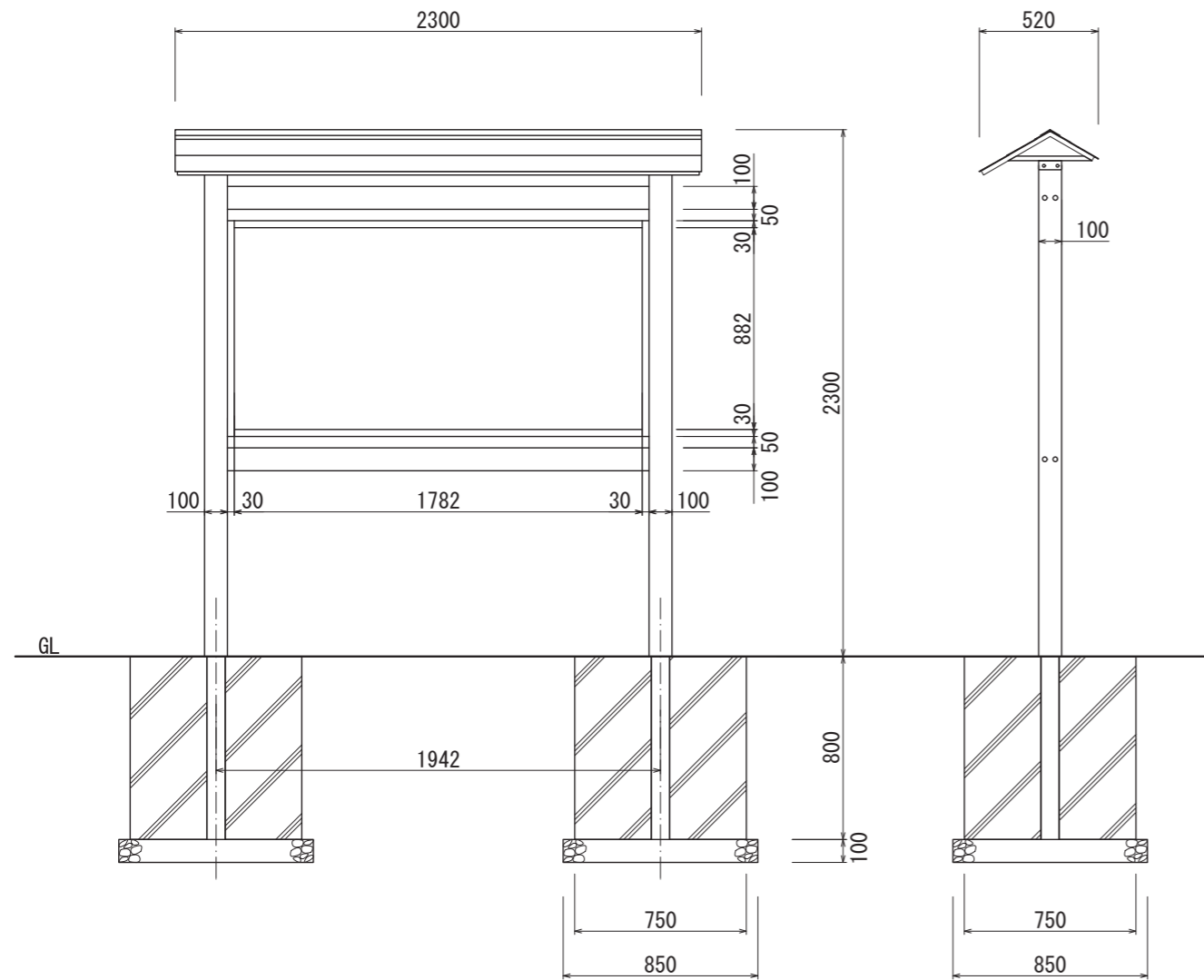
【正面図 S=1:30】
